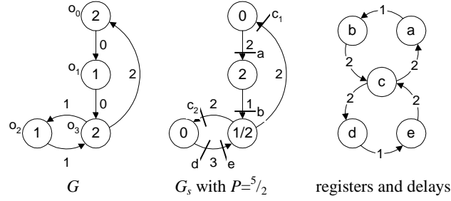
Fig. 8. k -periodic example
