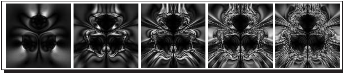
FIG. 5 – L'image fractale chaotique de l'erreur de modèle de la méthode d'Euler h = 0.1 (comparativement à la méthode d'Euler pour h = 0.01 ), pour une image de taille 128 \times 128 et pour respectivement t = 2 , t = 4 , t = 5 , t = 6 , t = 7 ( \approx 10 sec. de calcul).
