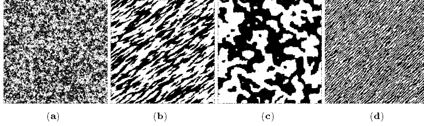
Fig. 2. Realizations of GD with specified parameters (see Table 1 for parameters values).
