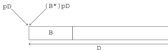
FIG. 9 – Conversion de pD , un pointeur sur un D , en un pointeur sur un B
